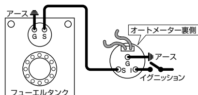
〔燃料計センサーユニット/オートメーター配線図〕
