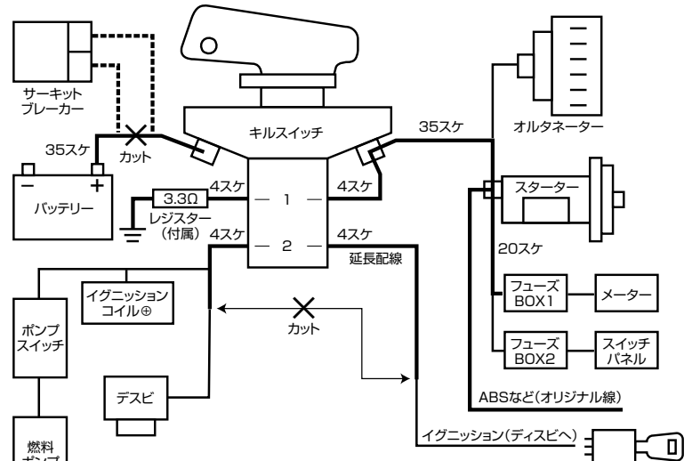
GE55 (配線図例)
