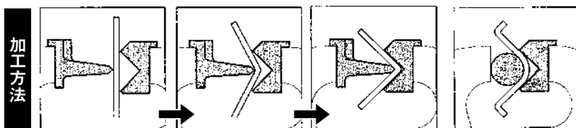
バイスを閉じて行き金属バーを90°まで曲げます。
