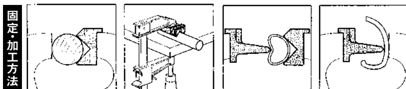
丸棒、パイプなどを固定。作業面に保持する。パイプの加工及び保持。変形した物の作成。
