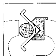
Vブロックと丸棒を使用してU字形を作成。
